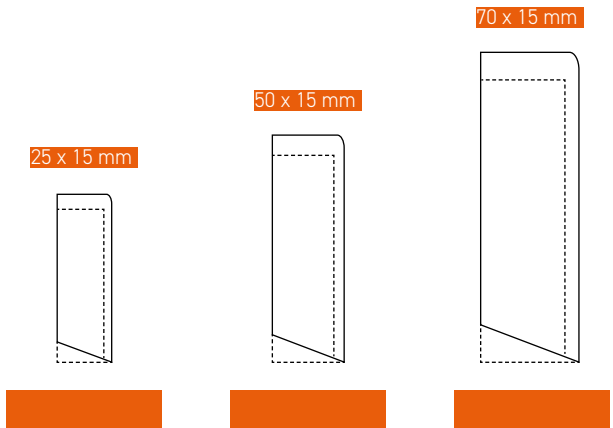
CUBE - IZDELANE PO NAROČILU
